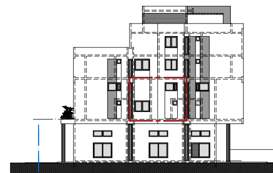
ELEVATION 2
